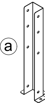
80874 Anclaje para arenero para colocar con pernos
